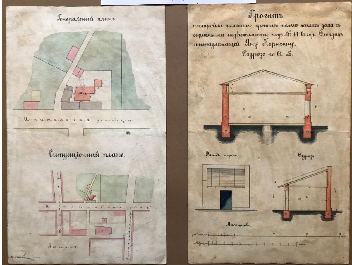
Fot. Projekt końcowy wykonany w 1911 r. przez jednego z pierwszych absolwentów Szkoły – Władysława Piątka.
